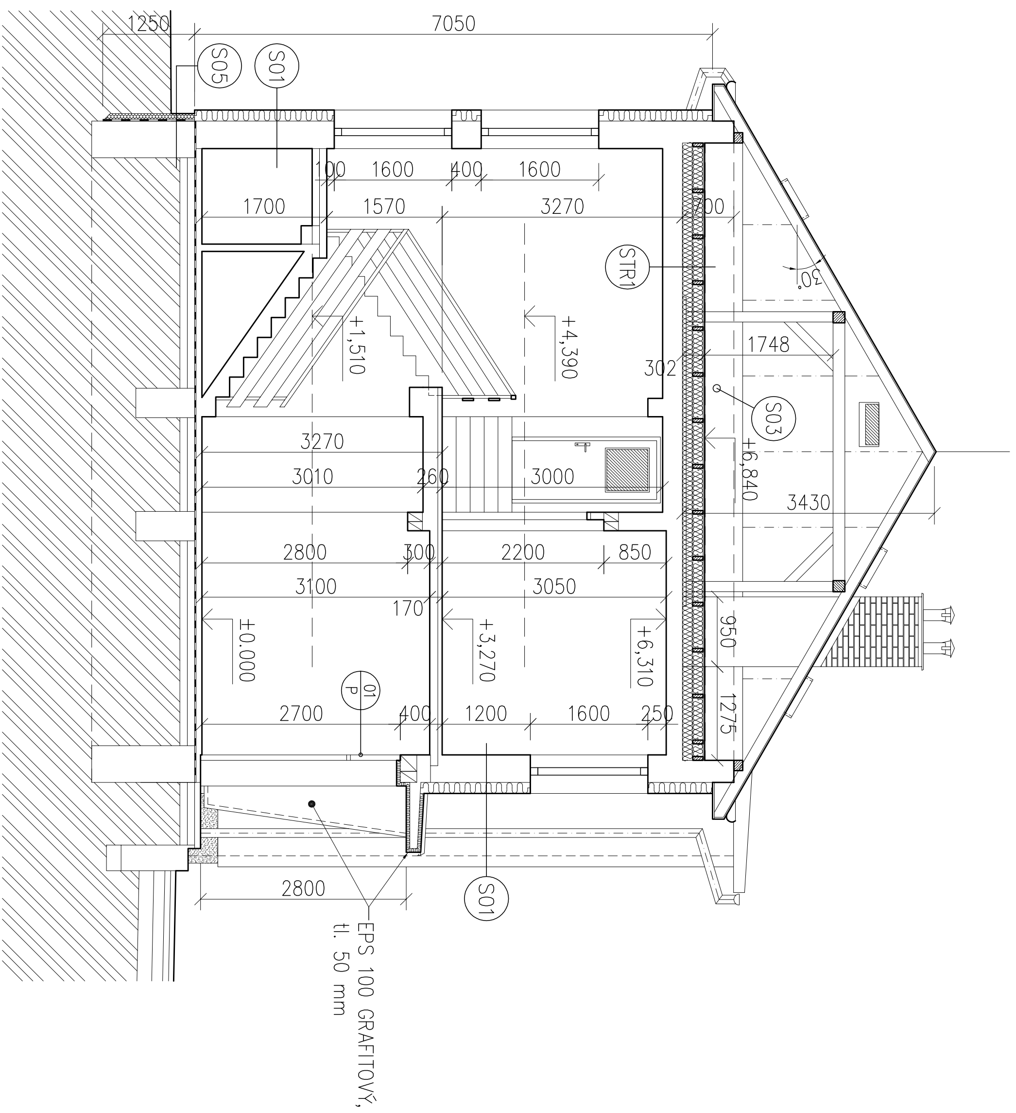
ŘEZ A-A – Navrhovaný stav
