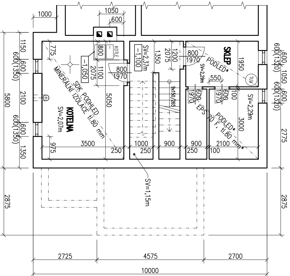
PŮDORYS SUTERÉNU – Stávající stav
