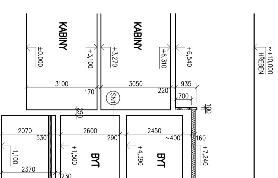
VÝŠKOVÉ ÚROVNĚ V MÍSTĚ ŘEZU B - SCHEMA M = 1:100
